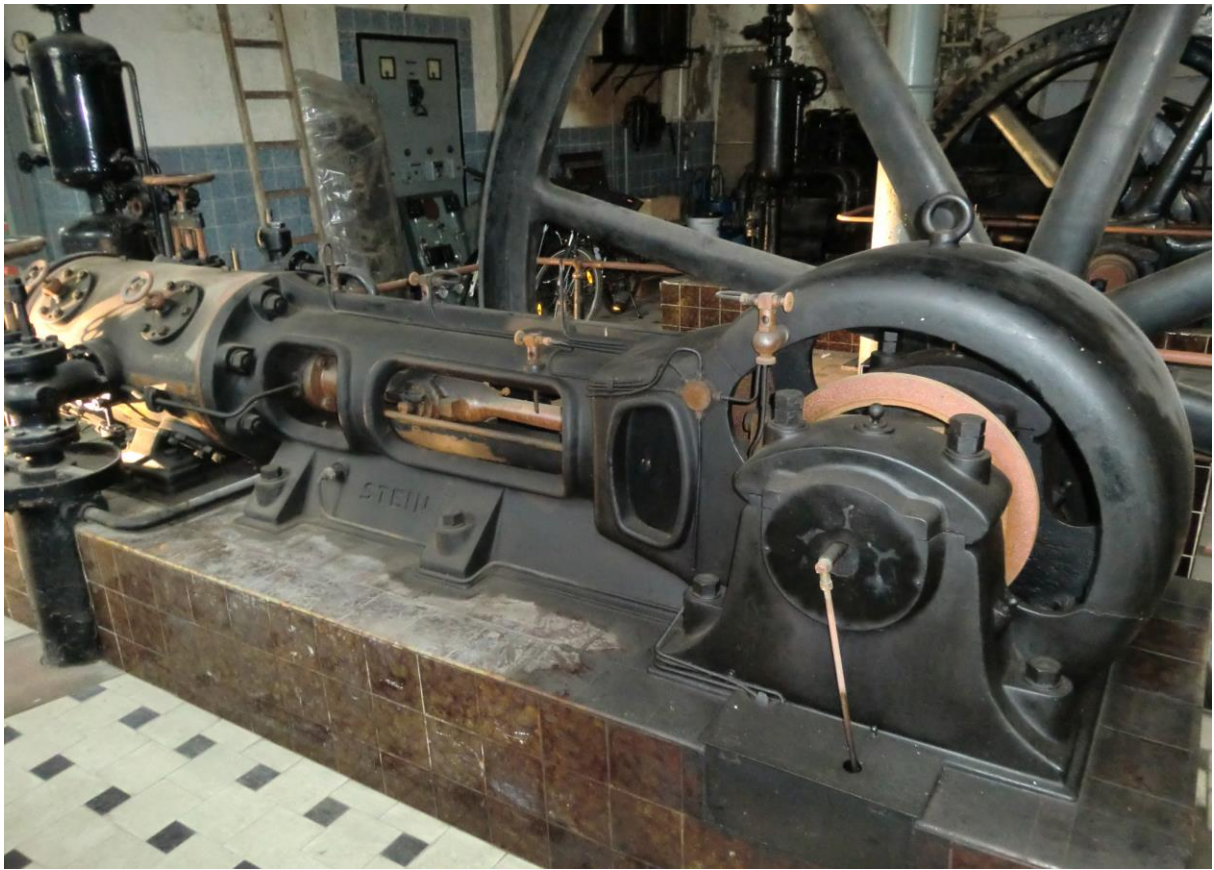
Verdichter der Firma Stein Bad Cannstadt
