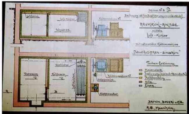
1901, die erste hermetisch gekapselte stopfbuchsenlose Kältemaschine der Welt (Patent Audifren Singrün). Was man damit u. a. kühlen konnte, zeigt hierzu die Projektzeichnung von BBC
